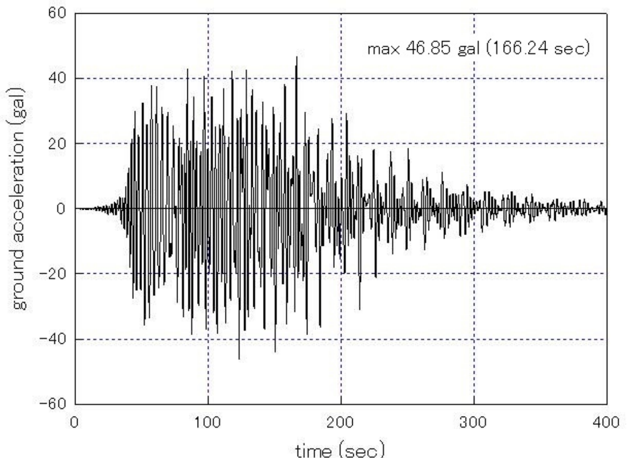
図 ka3-3.2.acceleration 地動加速度波形
