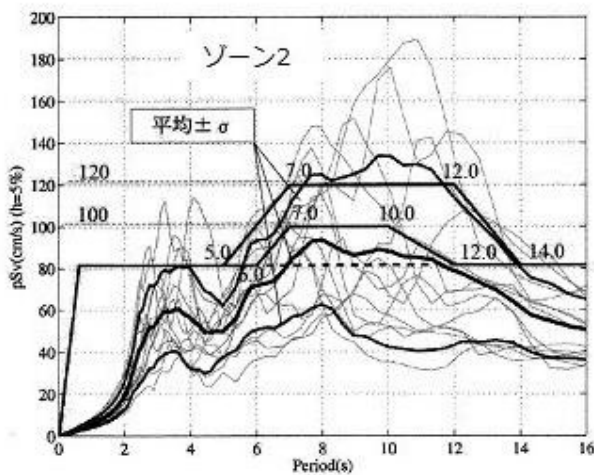
図 ka2.1.1 理論計算波の速度応答スペクトル
