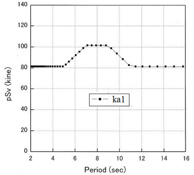
図 ka1.1.2 設計用速度応答スペクトル平均値
