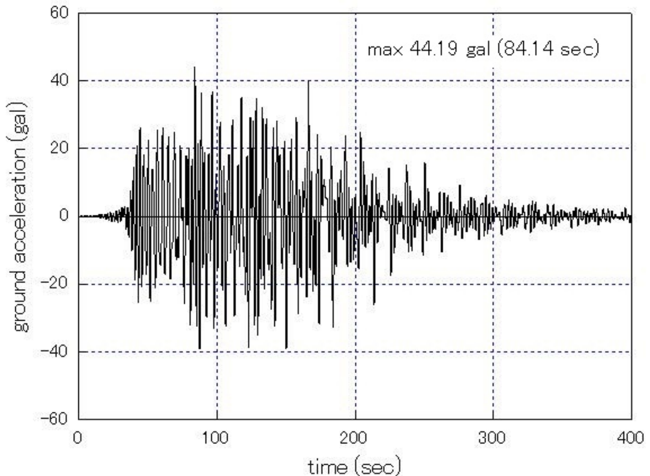
図 ka2-3.2.acceleration 地動加速度波形
