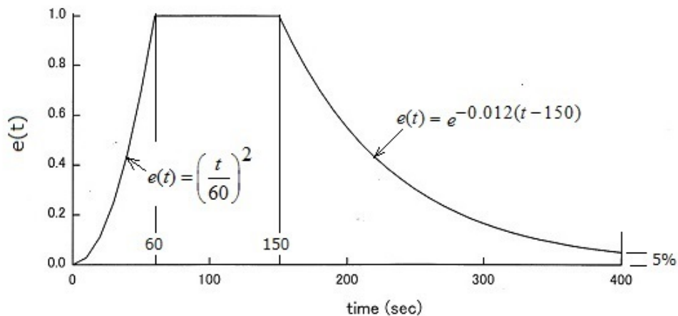
図 G-1 包絡曲線 Envelope-2
