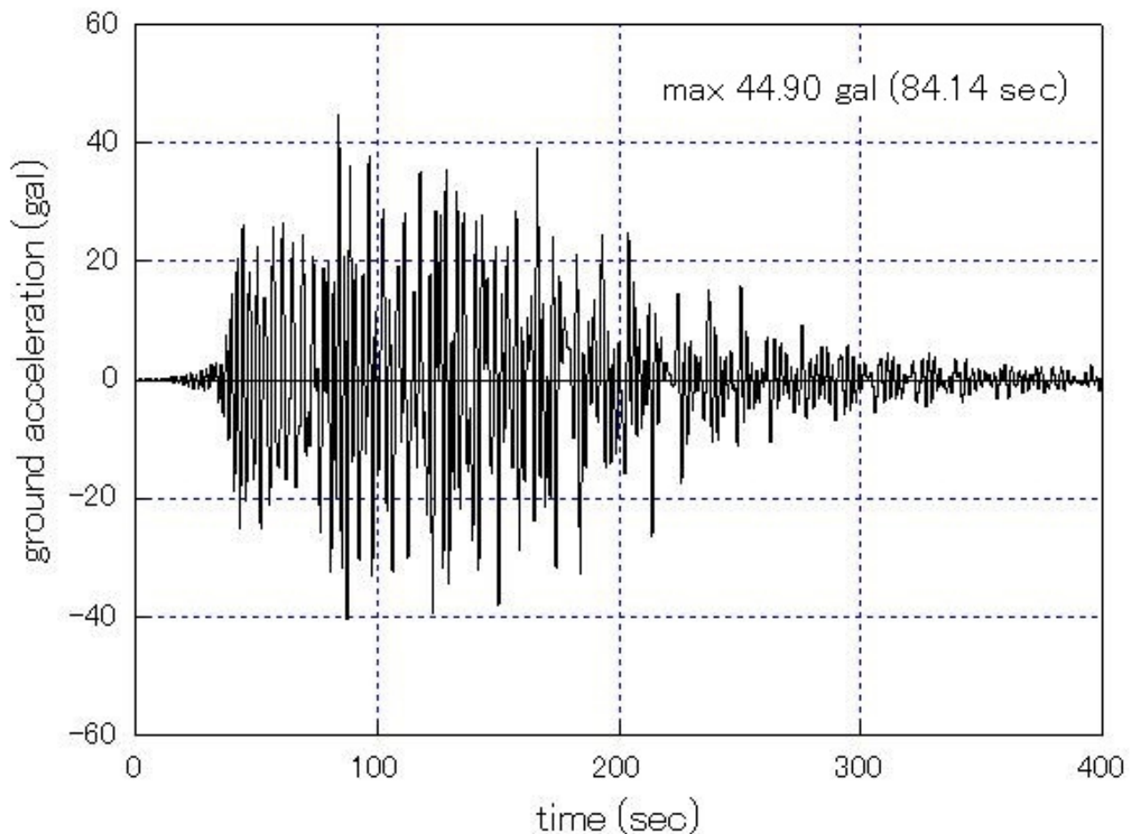
図 ka1-3.2.acceleration 地動加速度波形
