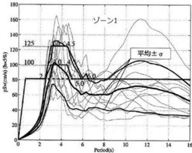
図 nb1.1.1 理論計算波の速度応答スペクトル
