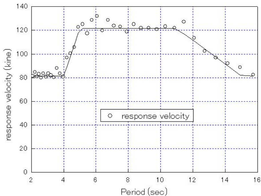
図 nb2.2.a 速度スペクトルの設計値と計算値の分布
