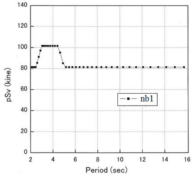
図 nb1.1.2 設計用速度応答スペクトル平均値
