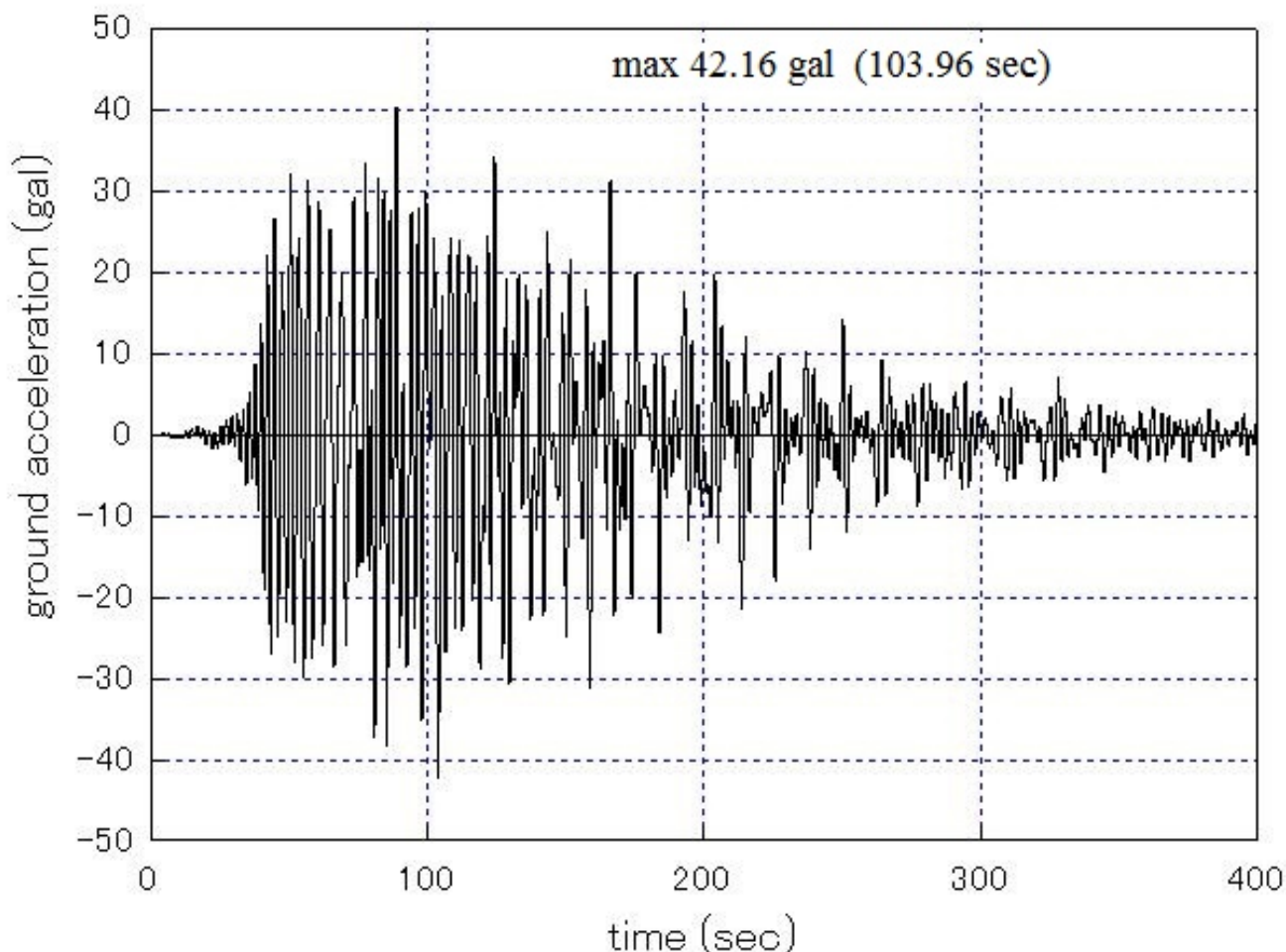
図 nb1-3.1.acceleration 地動加速度波形
