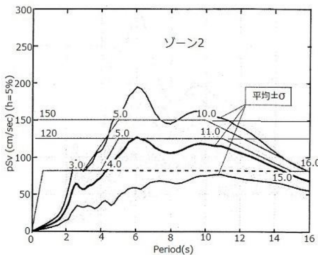
図 nb2.1.1 理論計算波の速度応答スペクトル
