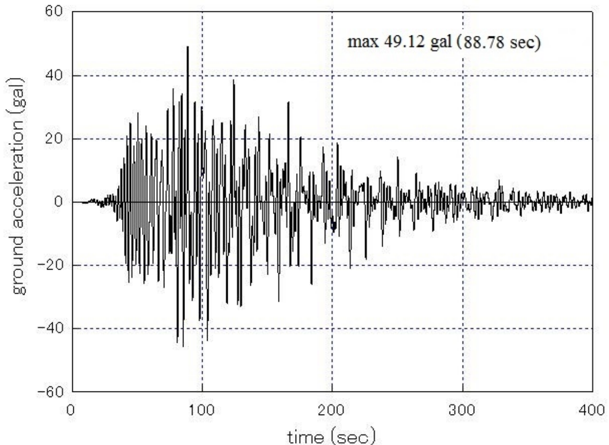
図 nb2-3.1.acceleration 地動加速度波形
