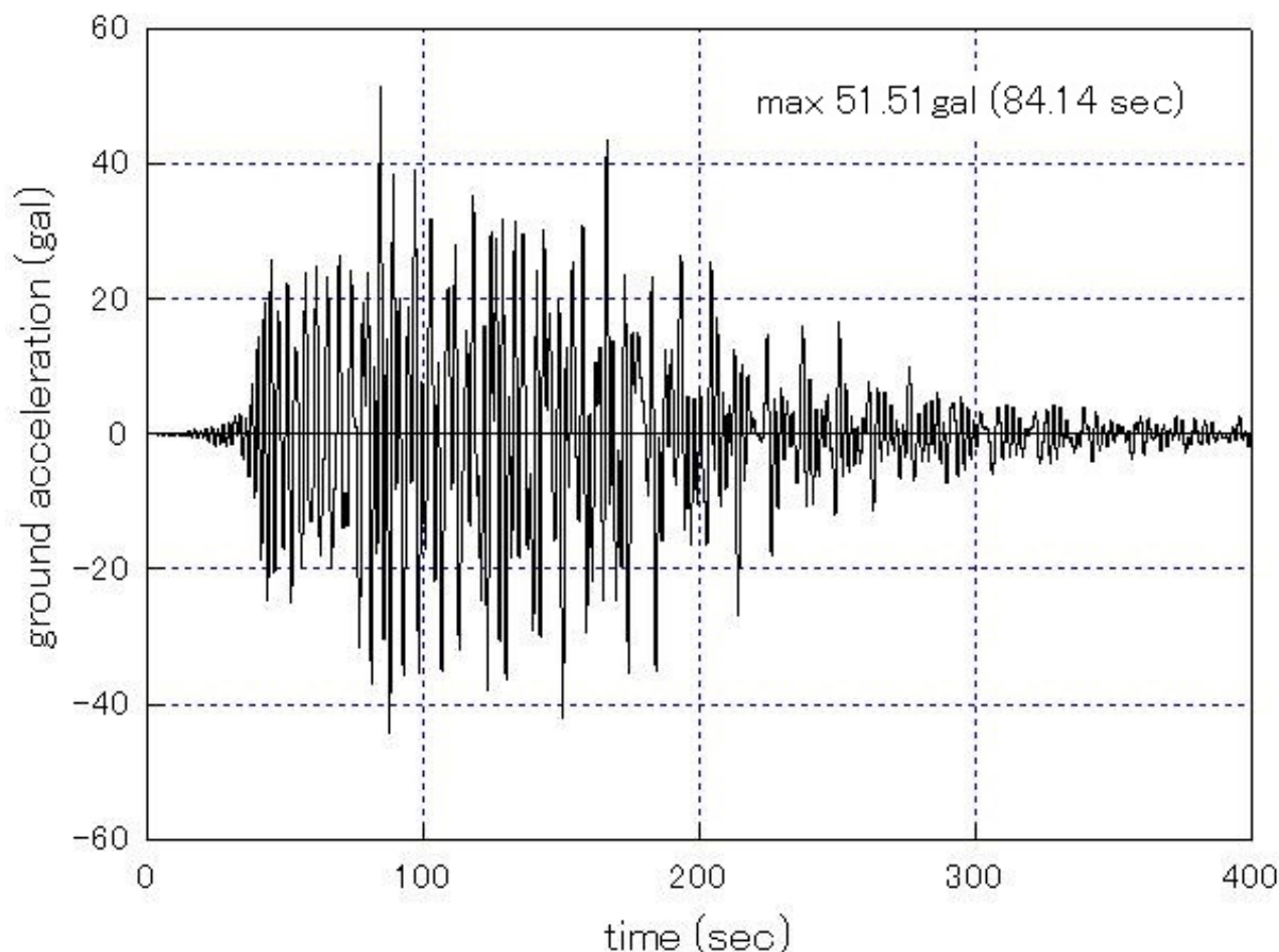
図 nb2-3.2.acceleration 地動加速度波形
