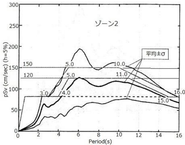
図nb2.1.1 理論計算波の速度応答スペクトル
