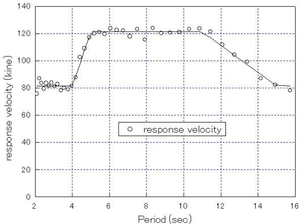
nb2.2.b 速度スペクトルの設計値と計算値の分布
