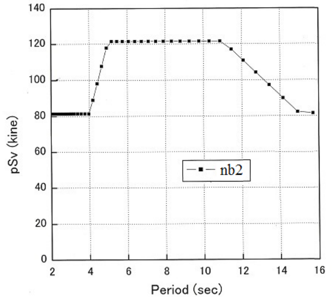
図 nb2.1.2 設計用速度応答スペクトル平均値
