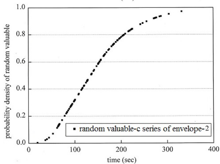
図 G-3 Envelope-2 の乱数分布状態
