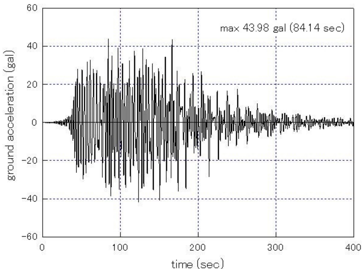
図 nb1-3.2.acceleration 地動加速度波形
