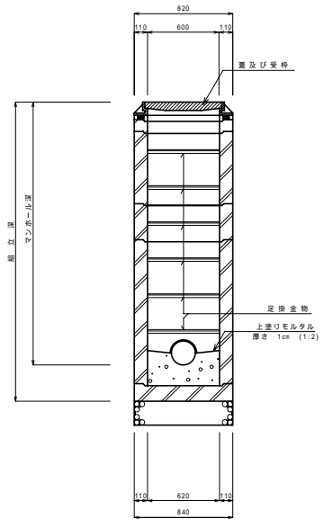
横断面図
