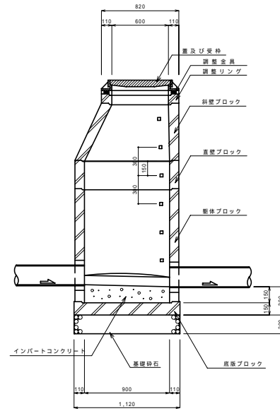
縦断面図
