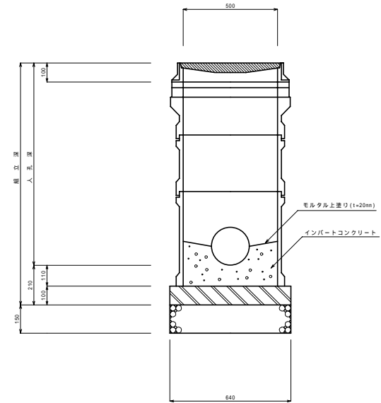
横断面図
