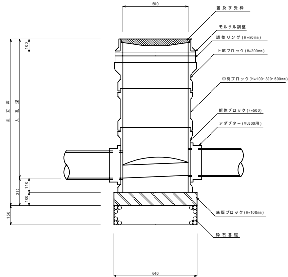
縦断面図
